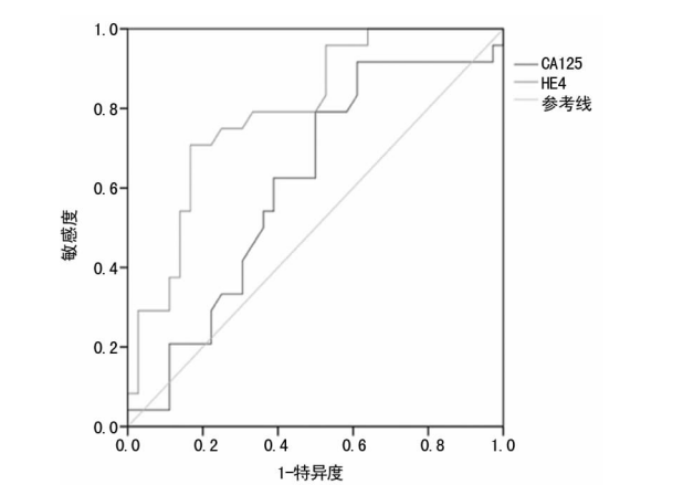
图 1 血清 HE4 与 CA125 诊断 EC 的 ROC 曲线
